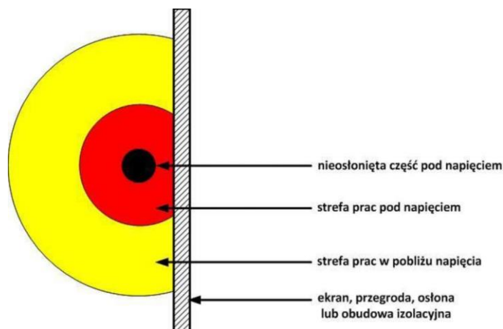
Rys.2 Ograniczenie minimalnego odstępu w powietrzu poprzez zastosowanie sprzętu ochronnego
